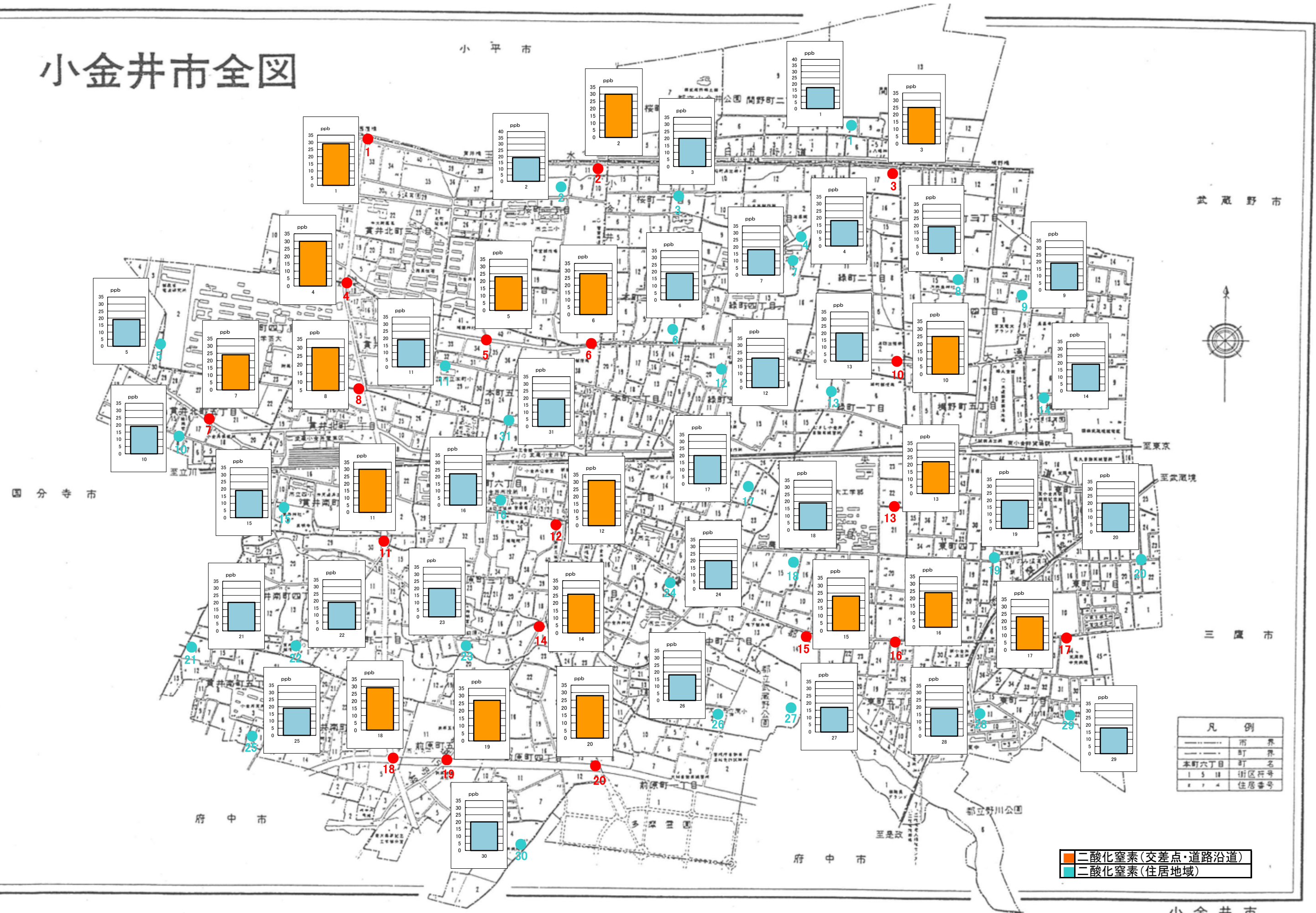
図5 二酸化窒素経年平均図(平成5年度～令和4年度)
