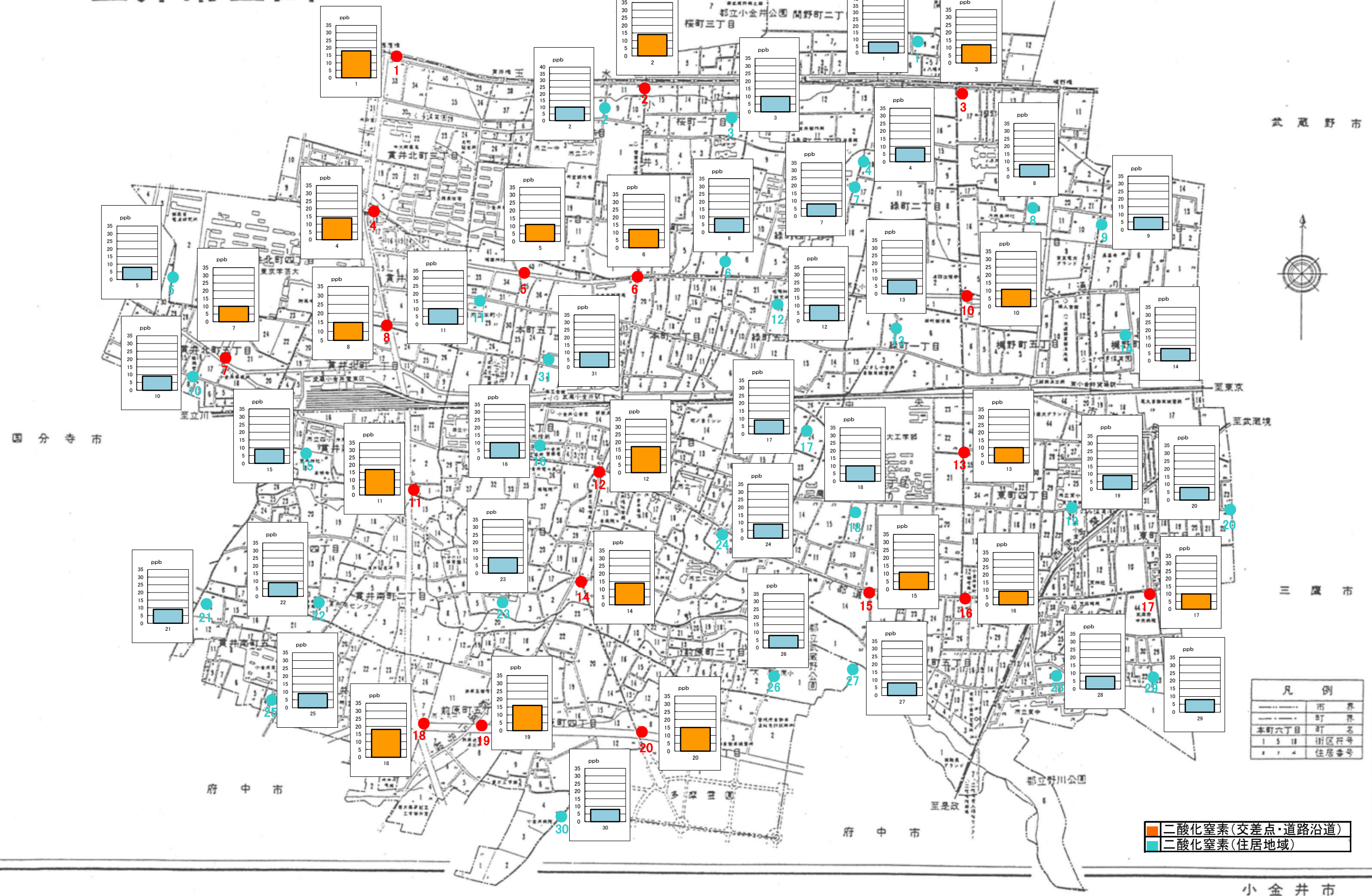
図2 二酸化窒素調査結果図(令和4年度)
