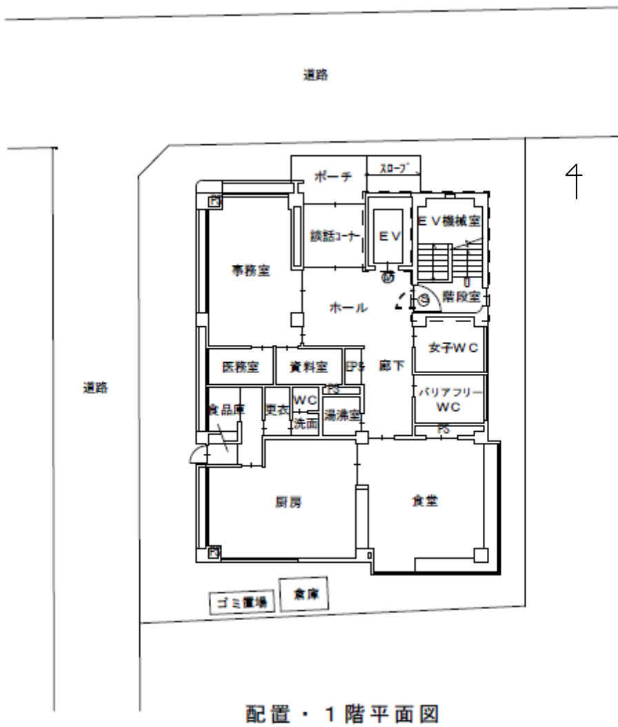
図 2-1 小金井市立本町高齢者在宅サービスセンターの施設配置（1階）
