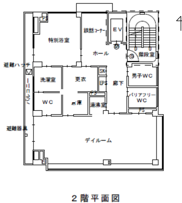
図 2-2 小金井市立本町高齢者在宅サービスセンターの施設配置（2階）
